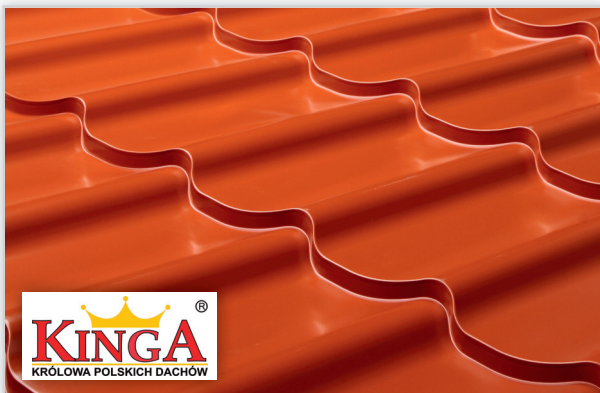
Blachodachówka Kinga. Ma klasyczny kształt imitujący tradycyjną dachówkę ceramiczną. Długość modułu [mm]: 350. Wysokość tloczenia [mm]: 20.
